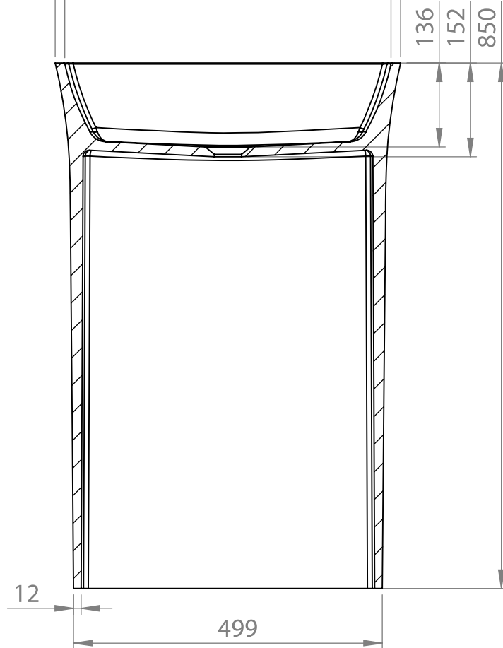
PRZEKRÓJ N-N SKALA 1 : 10
