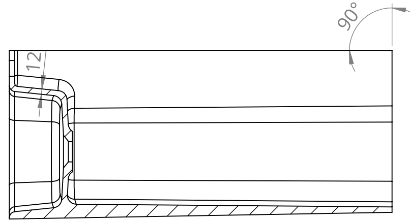
PRZEKRÓJ O-O SKALA 1 : 10
